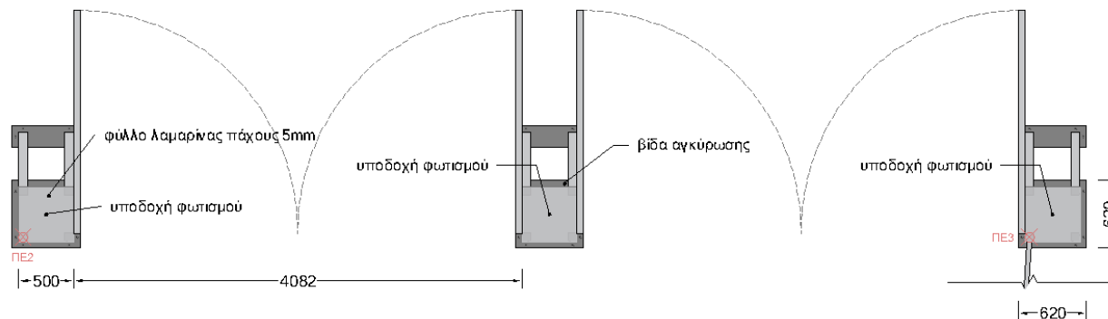
Εικόνα 22: Κάτοψη Πύλης 4
