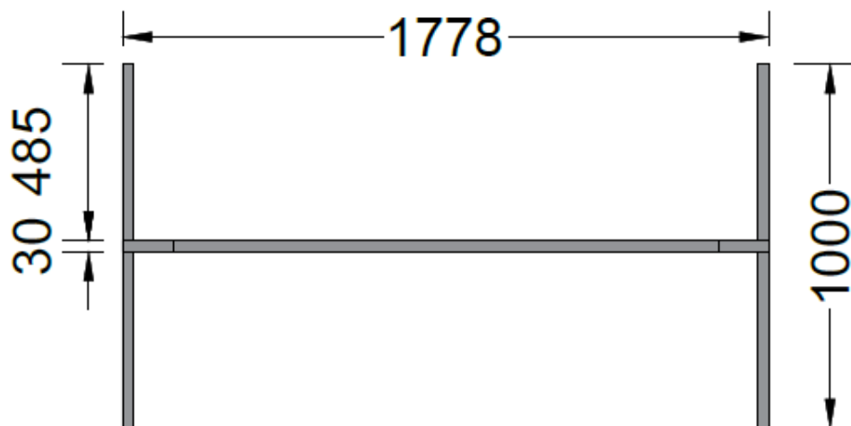
Εικόνα 11: Ενδεικτική κάτω όψη κινητής περίφραξης
