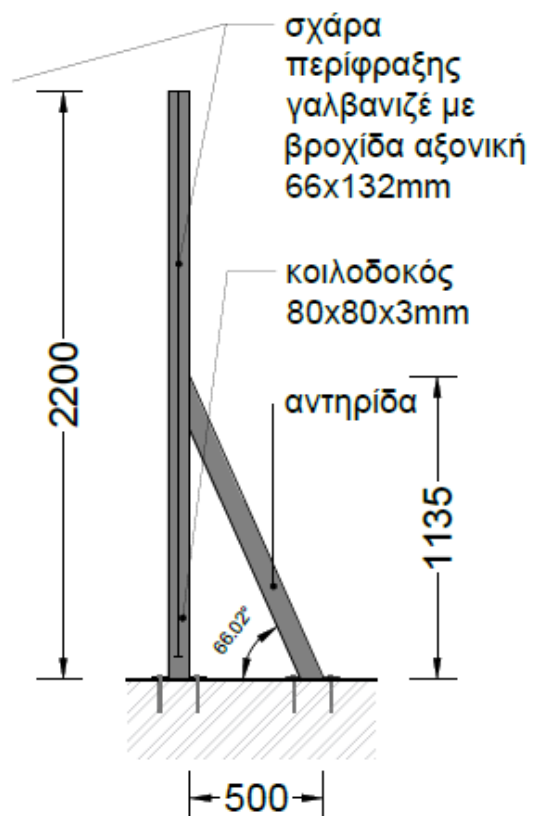
Εικόνα 3: Ενδεικτική πλάγια όψη περίφραξης ύψους 2,20μ.
