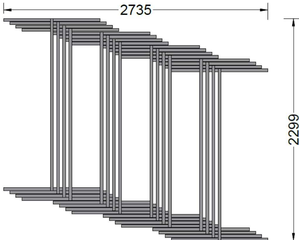
Εικόνα 16: Ενδεικτική κάτοψη διάταξης μονάδων κινητής περίφραξης
