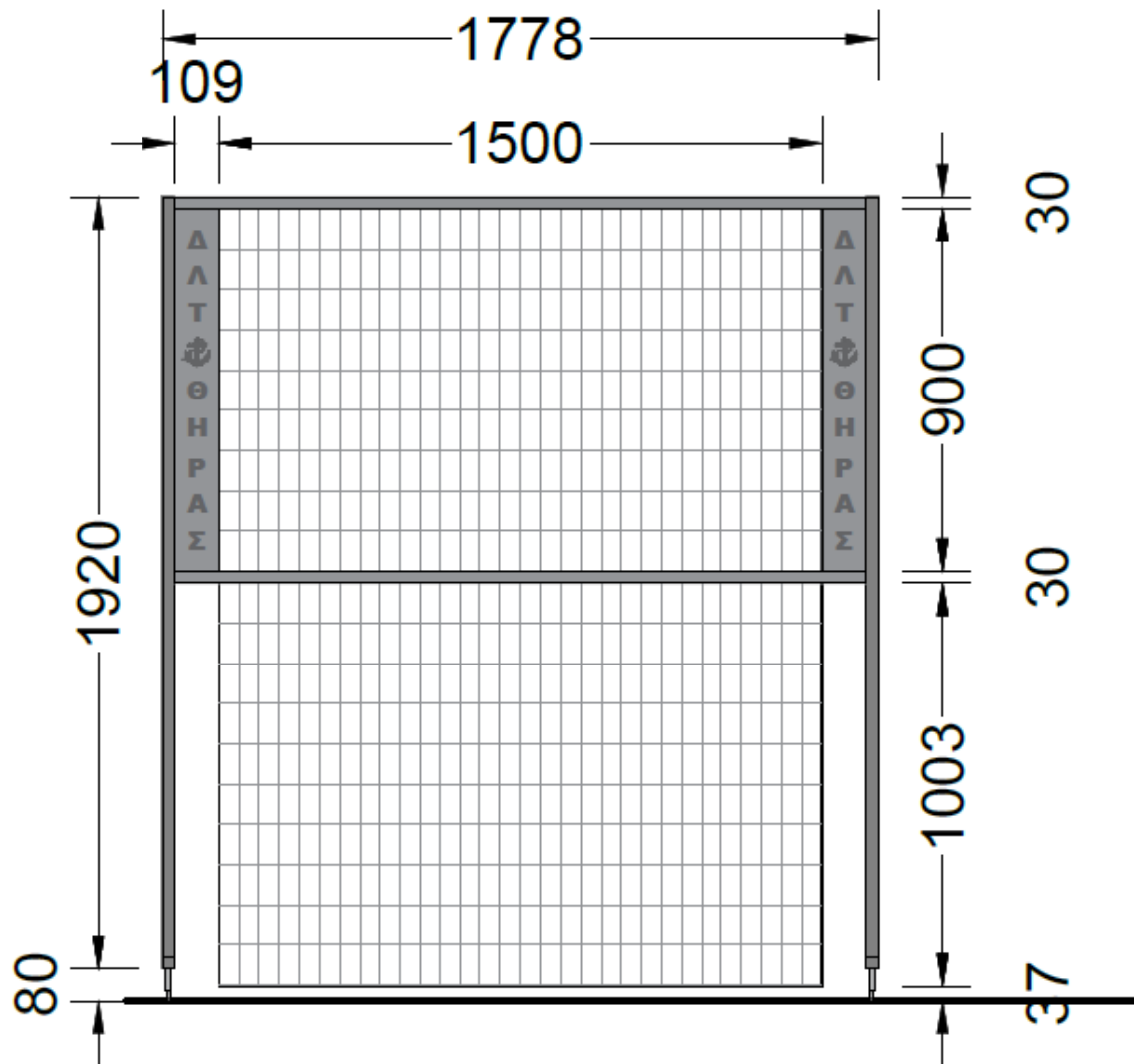
Εικόνα 10: Ενδεικτική όψη κινητής περίφραξης
