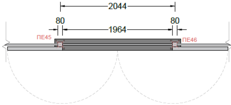
Εικόνα 30: : Κάτοψη Πύλης Διαφυγής
