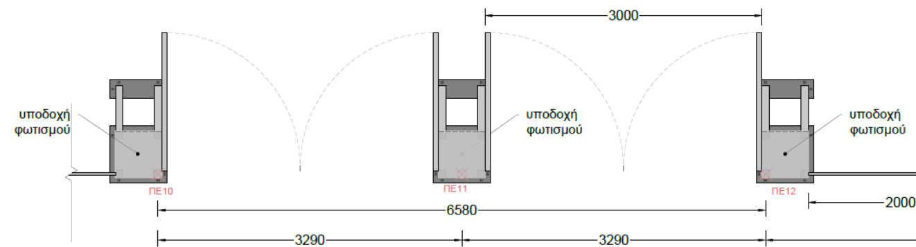
Εικόνα 25: Κάτοψη και Όψη Πύλης 2-3 ΠΕΖΩΝ
