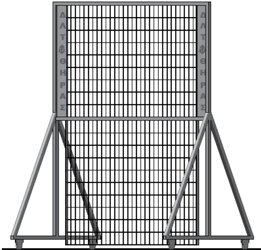
Εικόνα 13: Ενδεικτική τρισδιάστατη όψη κινητής περίφραξης
