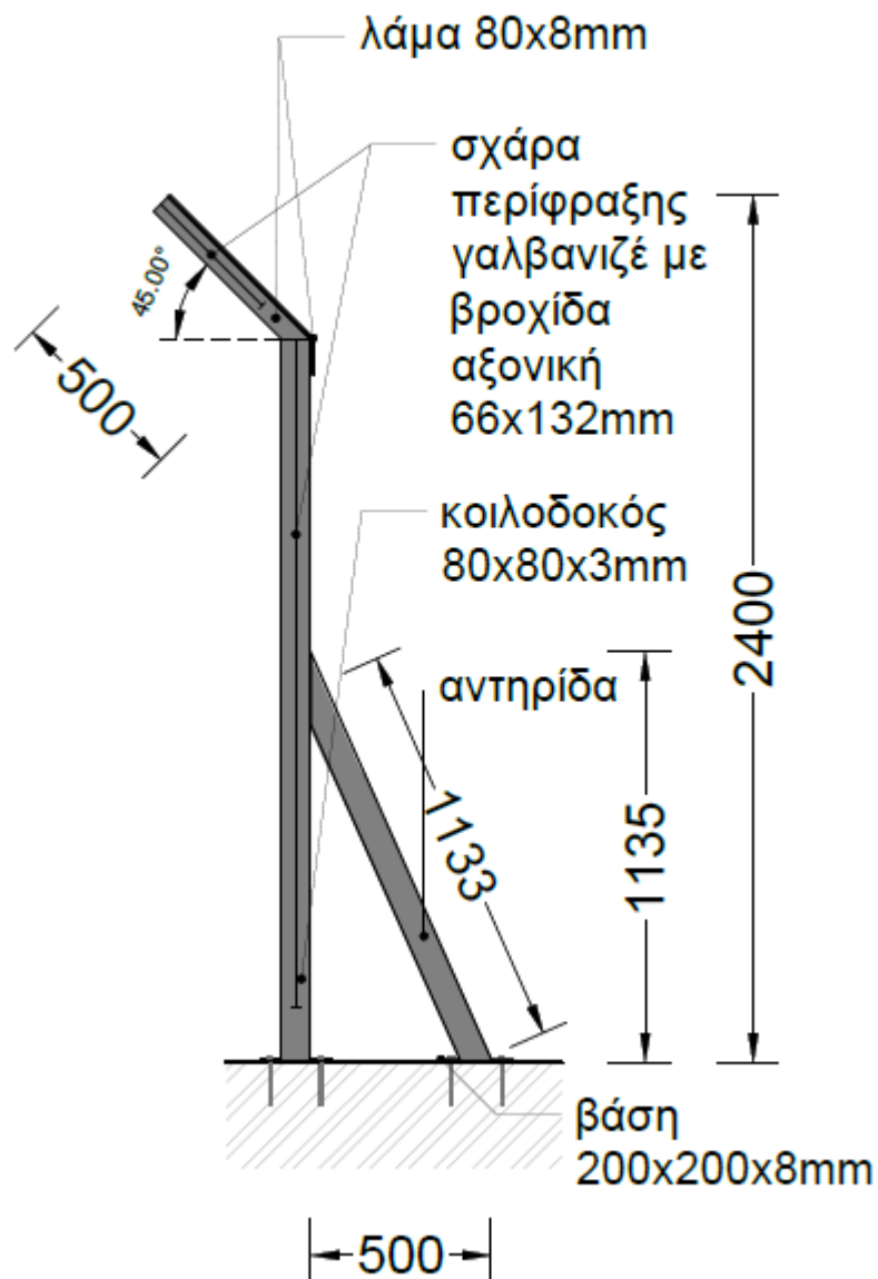
Εικόνα 6 Ενδεικτική πλάγια όψη περίφραξης ασφαλείας
