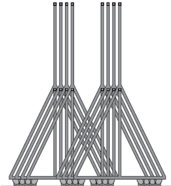
Εικόνα 14: Ενδεικτική πλάγια όψη διάταξης μονάδων κινητής περίφραξης
