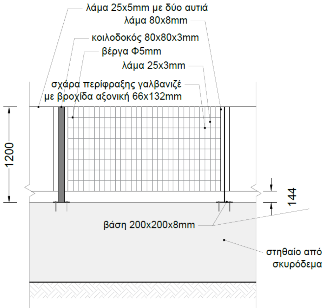
Εικόνα 7: Ενδεικτική όψη περίφραξης ύψους 1,20μ. επί στηθαίου
