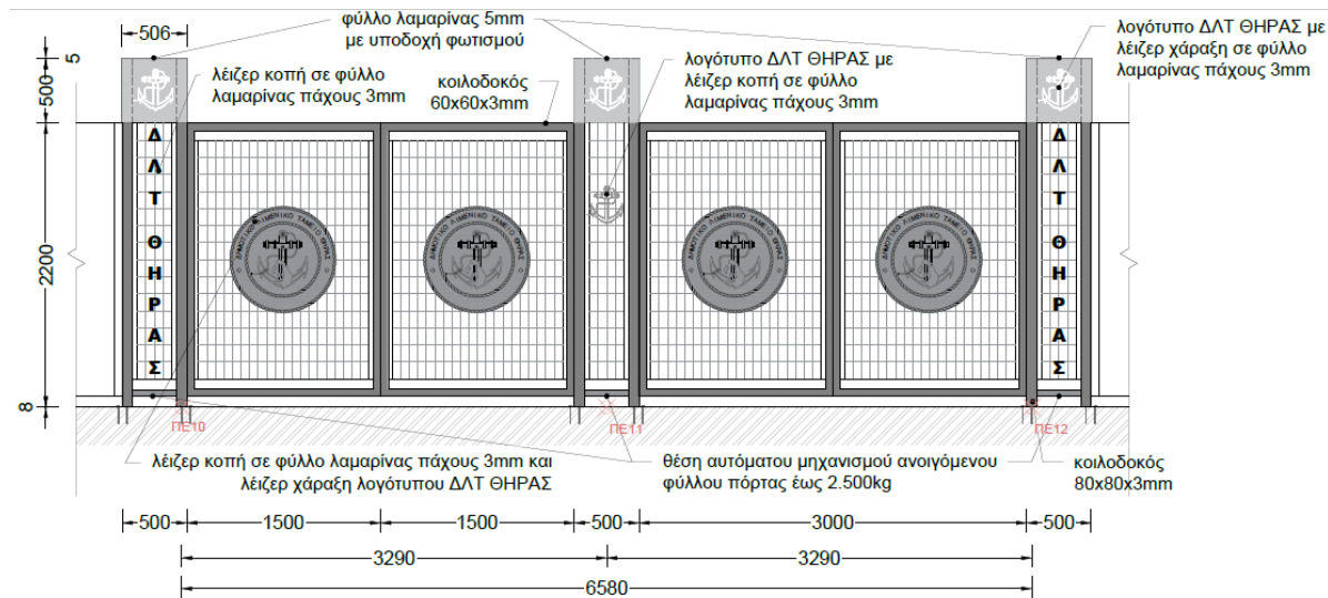
Εικόνα 24: Όψη Πύλης 2-3 ΠΕΖΩΝ
