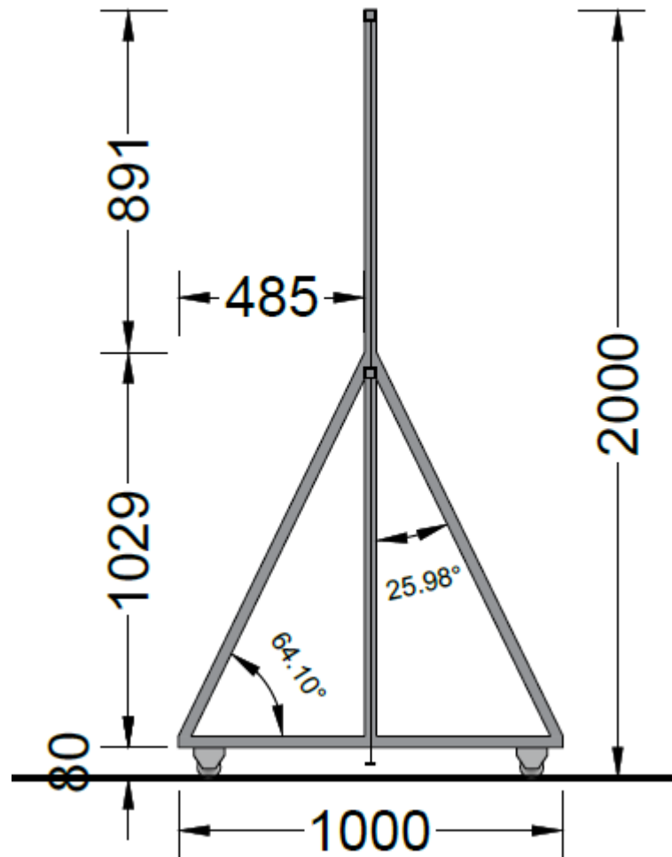
Εικόνα 12: Ενδεικτική πλάγια όψη κινητής περίφραξης
