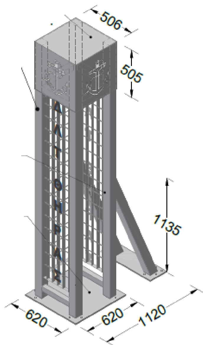
Εικόνα 20: Ενδεικτικό τρισδιάστατο σχέδιο τετράδας ορθοστατών που λειτουργεί ως άξονας των θυρών.
