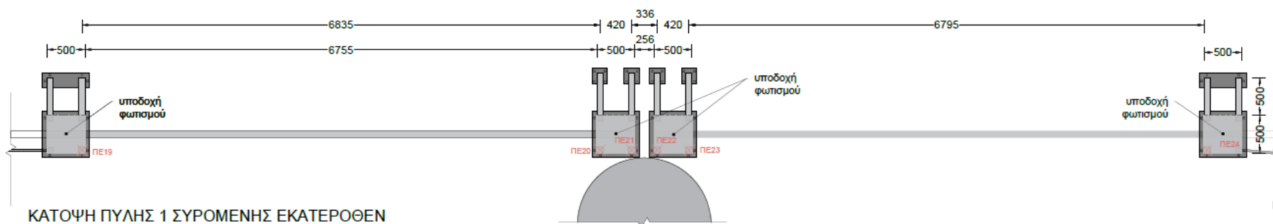
Εικόνα 26: Κάτοψη, πλάγια όψη και Όψη Πύλης 1
