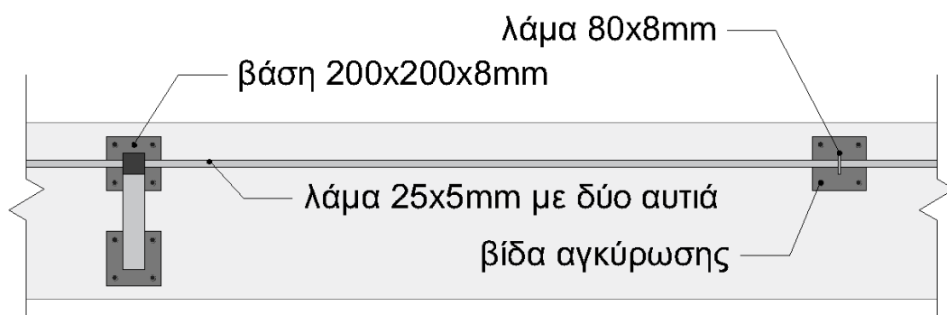
Εικόνα 8: Ενδεικτική κάτοψη περίφραξης ύψους 1,20μ. επί στηθαίου
