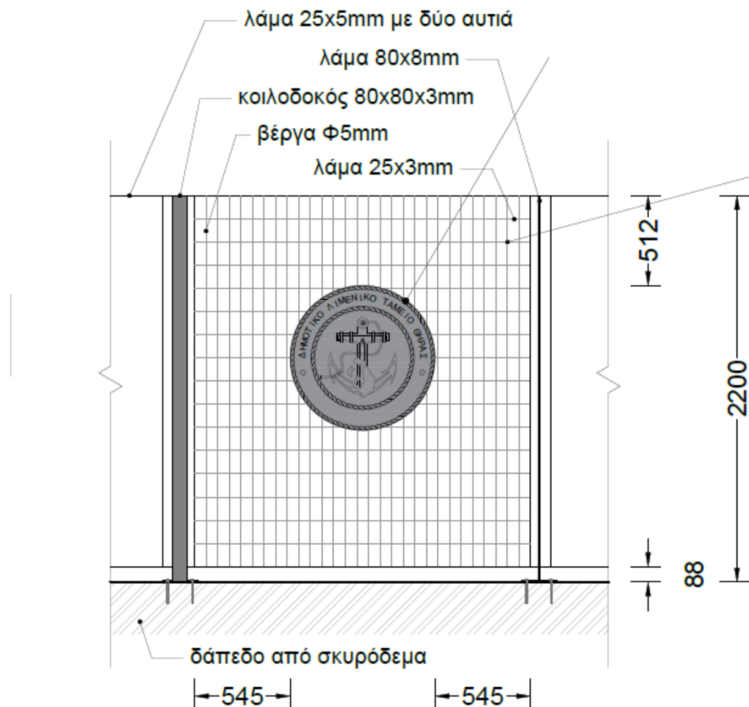
Εικόνα 1: Ενδεικτική όψη περίφραξης ύψους 2,20μ.
