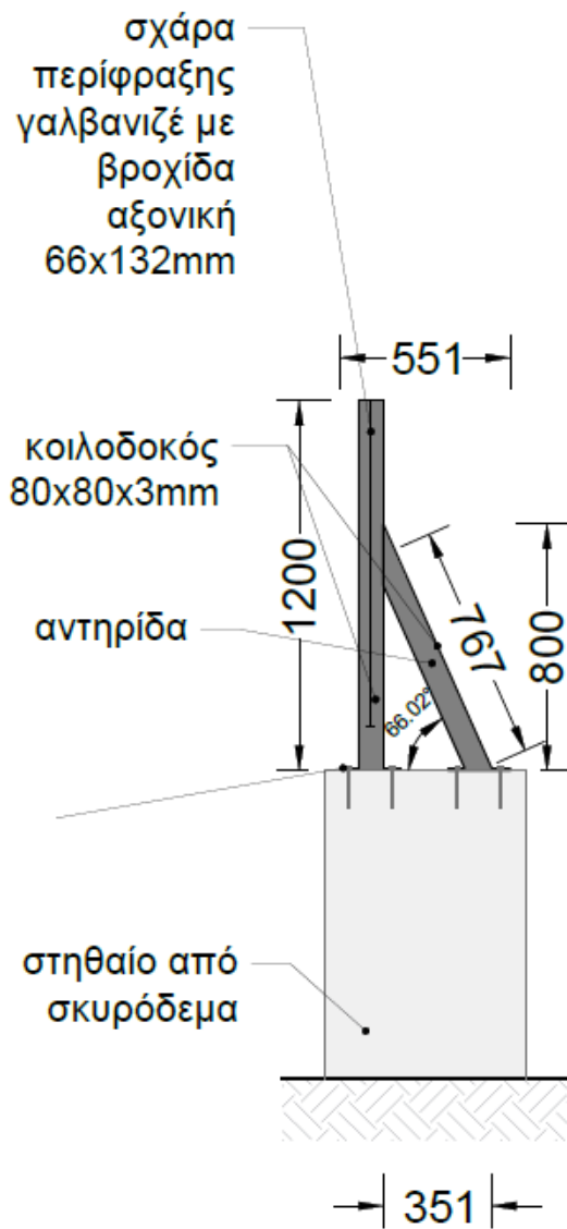
Εικόνα 9: Ενδεικτική πλάγια όψη περίφραξης επί στηθαίου
