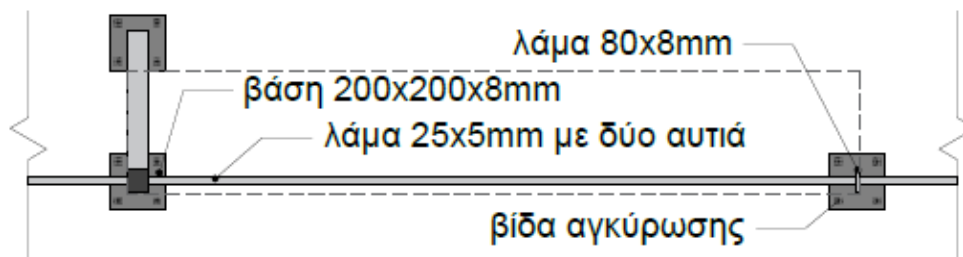
Εικόνα 5: Ενδεικτική κάτοψη περίφραξης ασφαλείας
