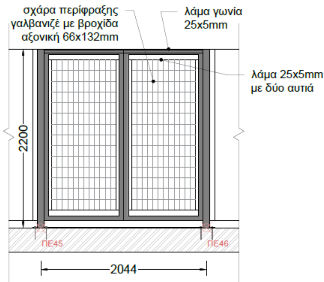
Εικόνα 29: Όψη Πύλης Διαφυγής
