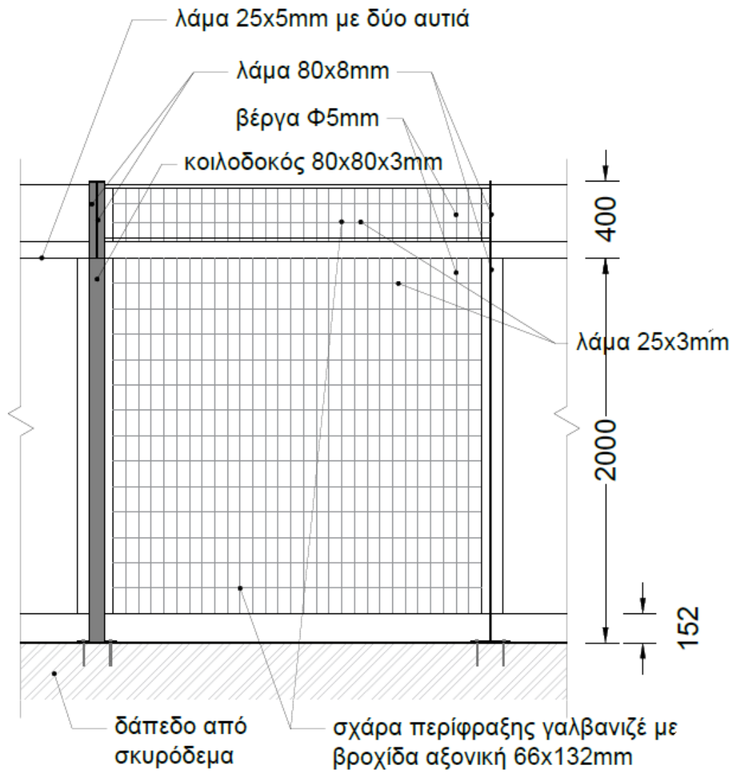
Εικόνα 4: Ενδεικτική όψη περίφραξης ασφαλείας ύψους 1μ
