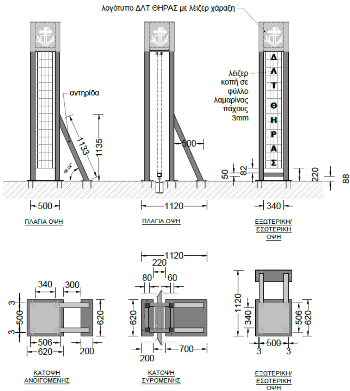
Εικόνα 19:Ενδεικτικές πλάγιες όψεις και κατόψεις τετράδας ορθοστατών για ανοιγόμενες και συρόμενες πύλες
