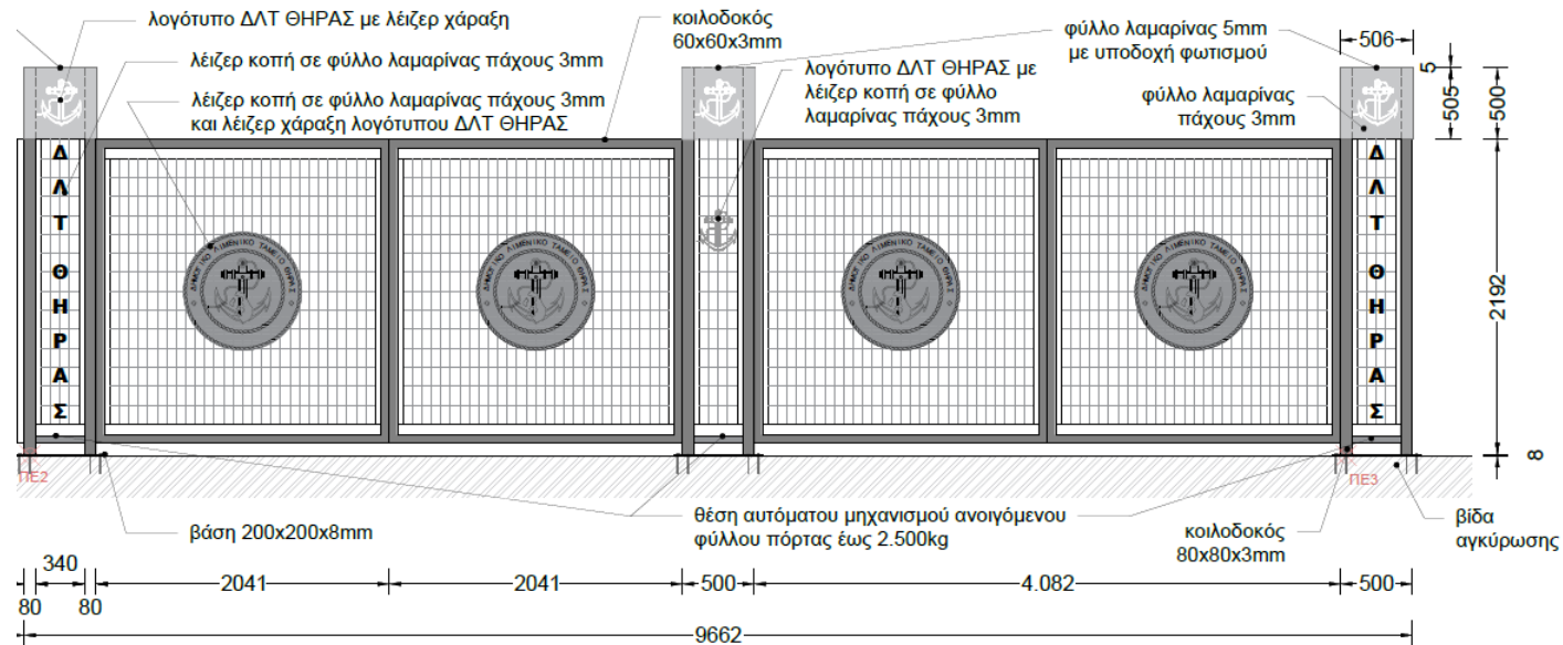
Εικόνα 21: Πρόσοψη Πύλης 4
