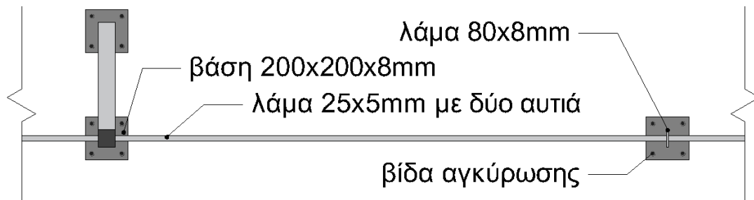
Εικόνα 2: Ενδεικτική κάτοψη περίφραξης ύψους 2,20μ.
